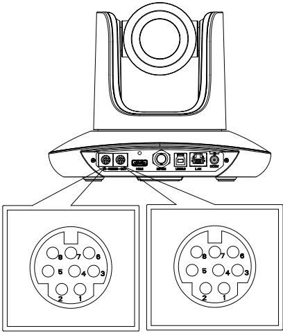
VISCA IN & Mini DIN Connection
